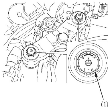
(1) Регулятор предварительного сжатия пружины
